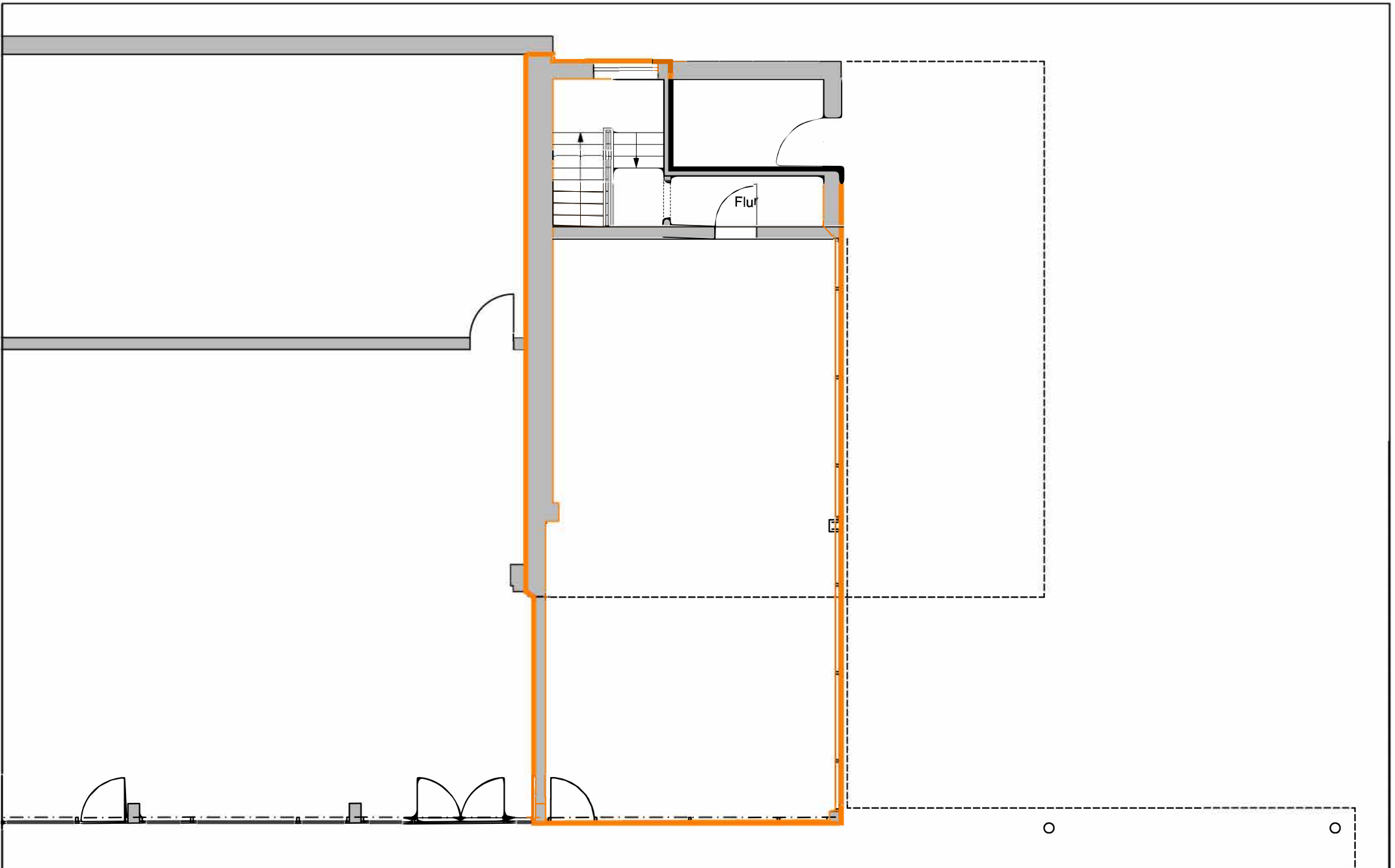
Hamburg, EKZ Manshardtstraße Grundriss Erdgeschoss (Grundriss Teilbereich)
