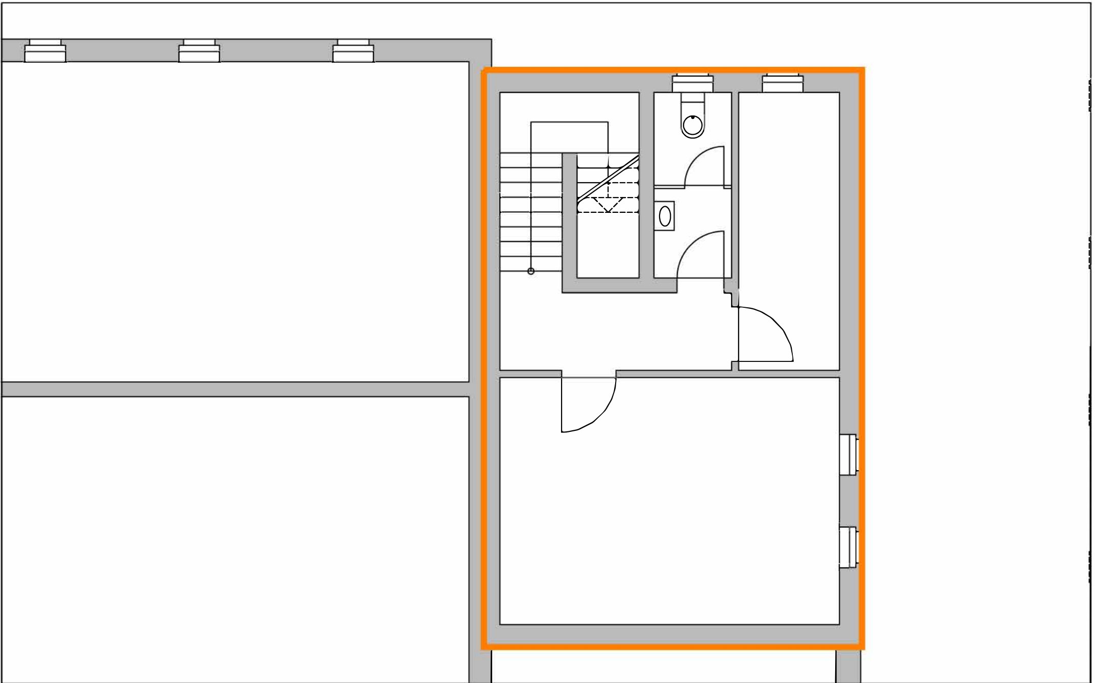
Hamburg, EKZ Manshardtstraße Grundriss Kellergeschoss (Teilbereich)
